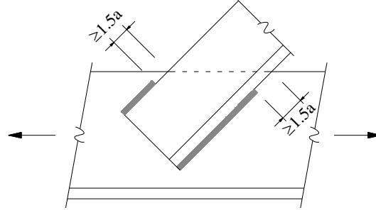
Şekil 13.6 – Çekme etkisindeki bir elemana köşe kaynaklı bağlantı
