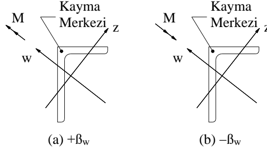
Şekil 9.2 – Eğilme momenti etkisindeki farklı kollu korniyerler için \beta_w işareti tanımı
